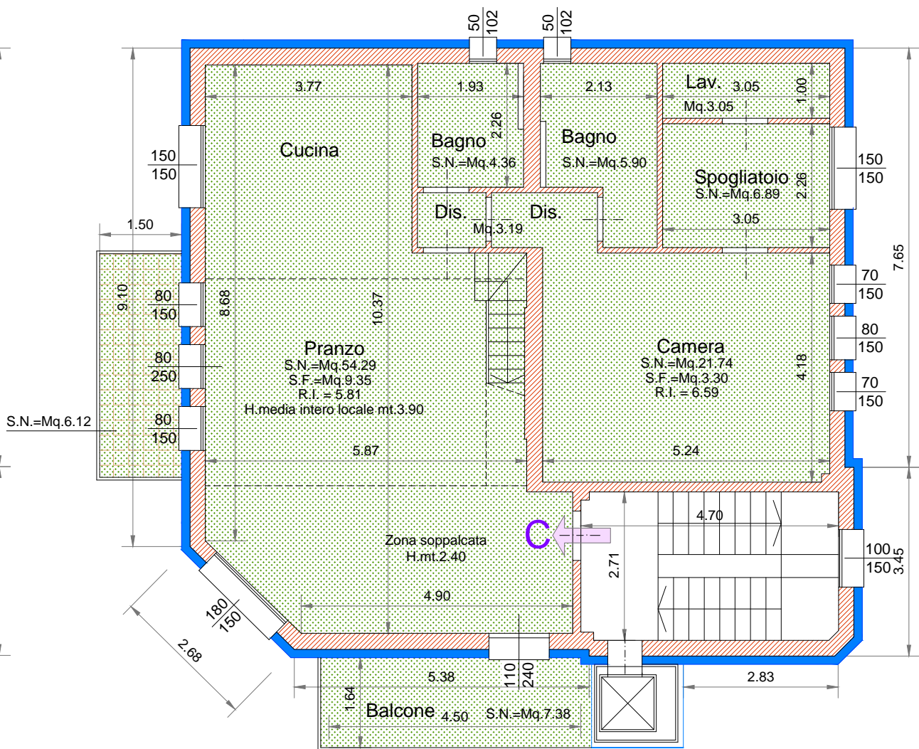
PIANTA PIANO SECONDO H.mt.2.95
